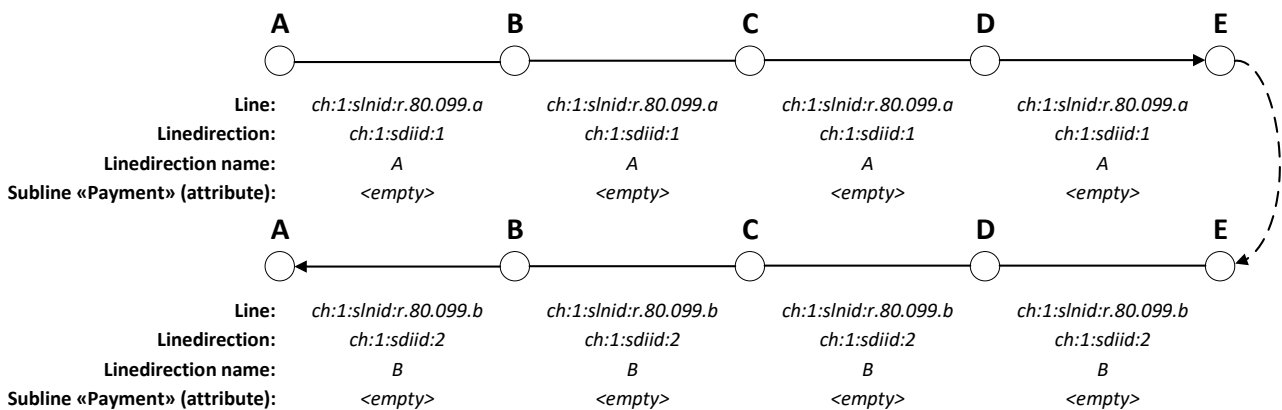
Abbildung 12: Beispiel zur Verwendung einer technischen Teillinie.
